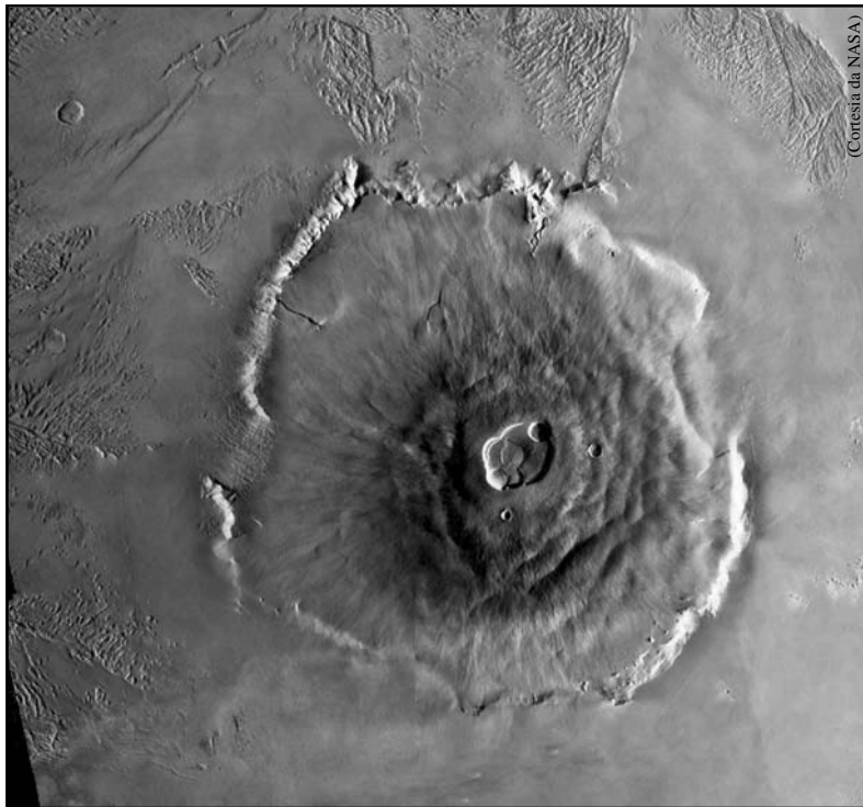
Figura 7: Monte Olimpus.
