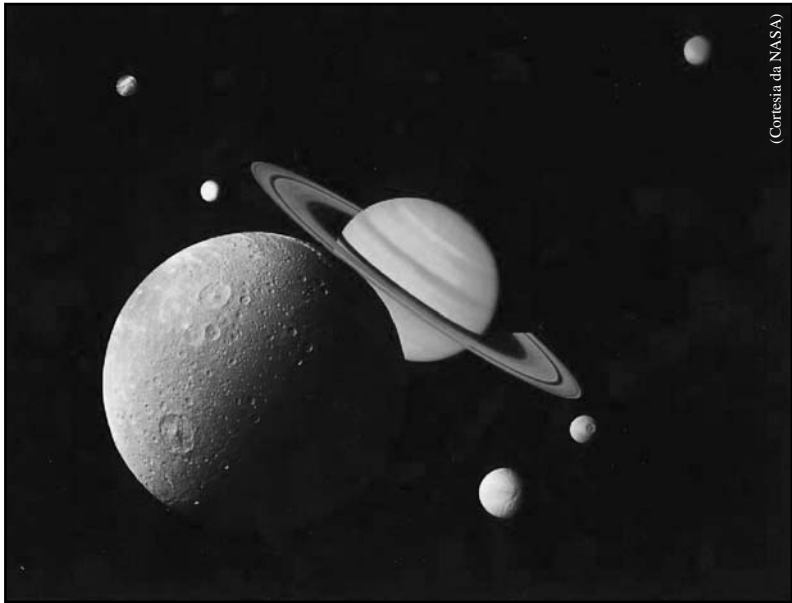
Figura 11: Planeta Saturno.
