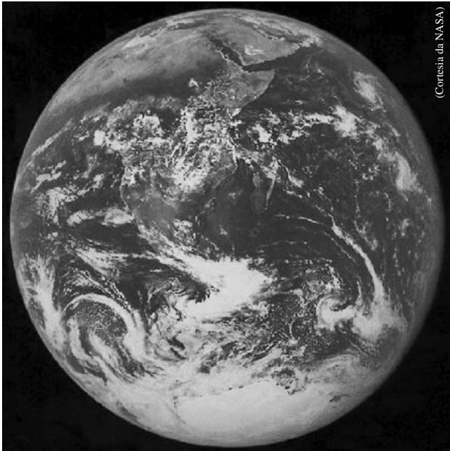
Figura 28: Planeta Terra.
