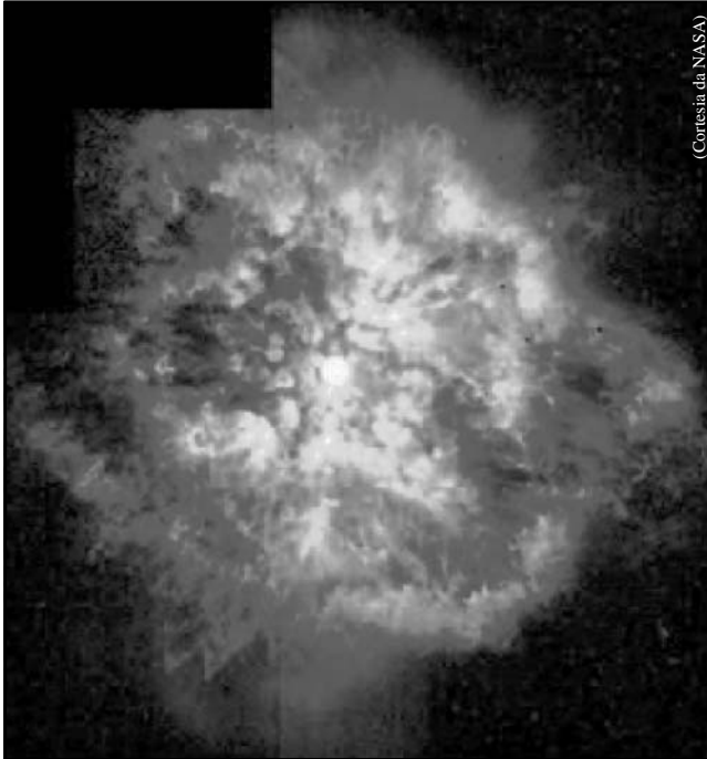
Figura 22: Estrela WR124.
